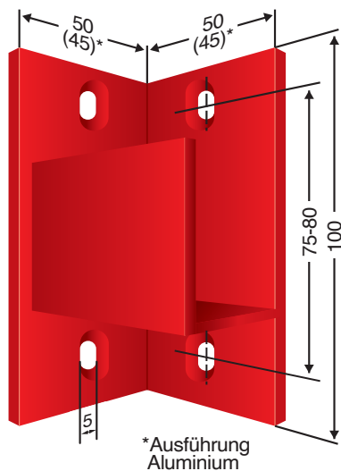
Balken-Halter
